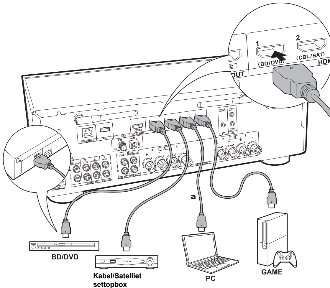
a HDMI-kabel
